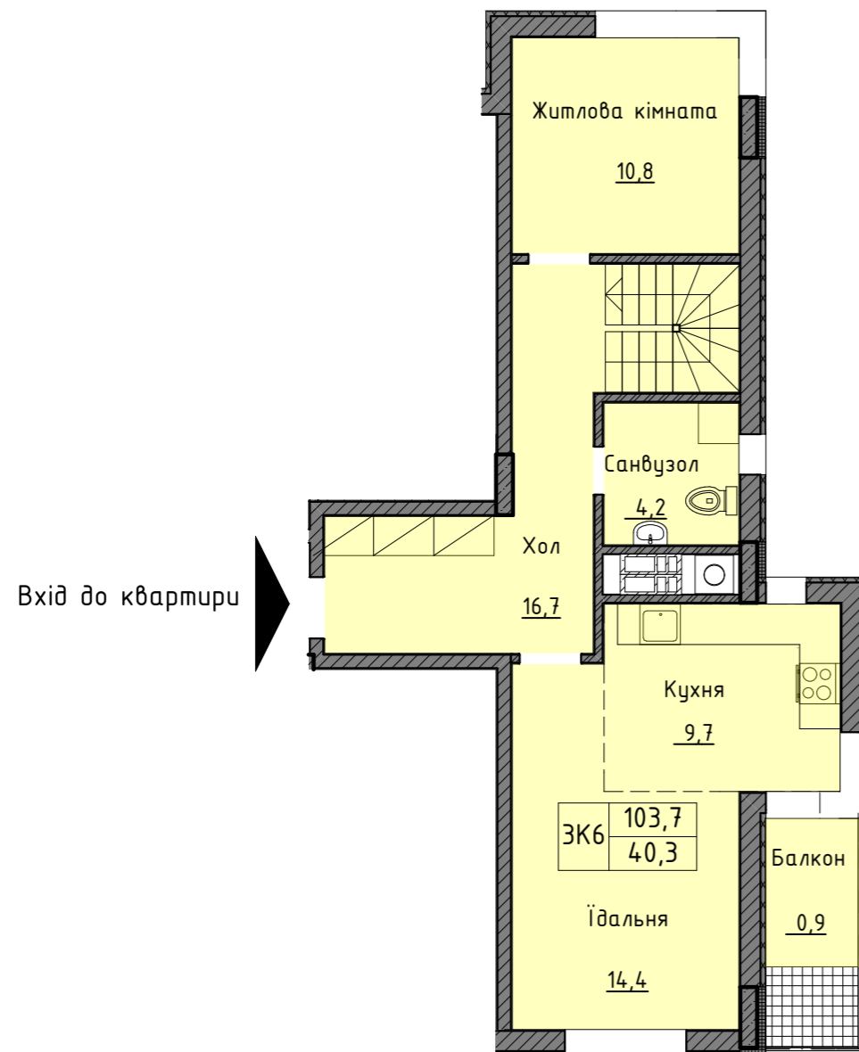
План квартири нижній рівень
